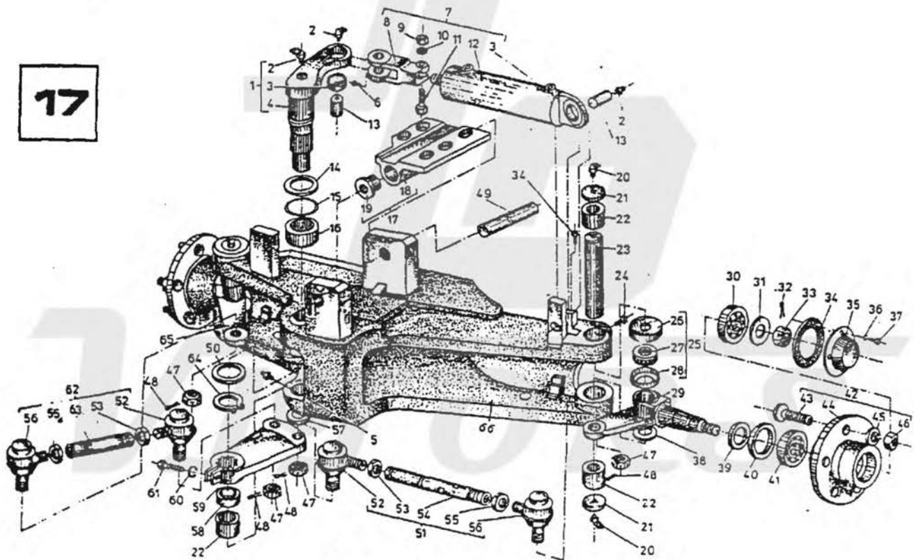
УПРАВЛЯЕМЫЙ МОСТ (в сборе) Управляемый мост
