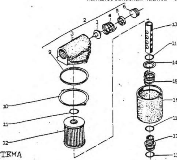
Фильтр гидравлический
