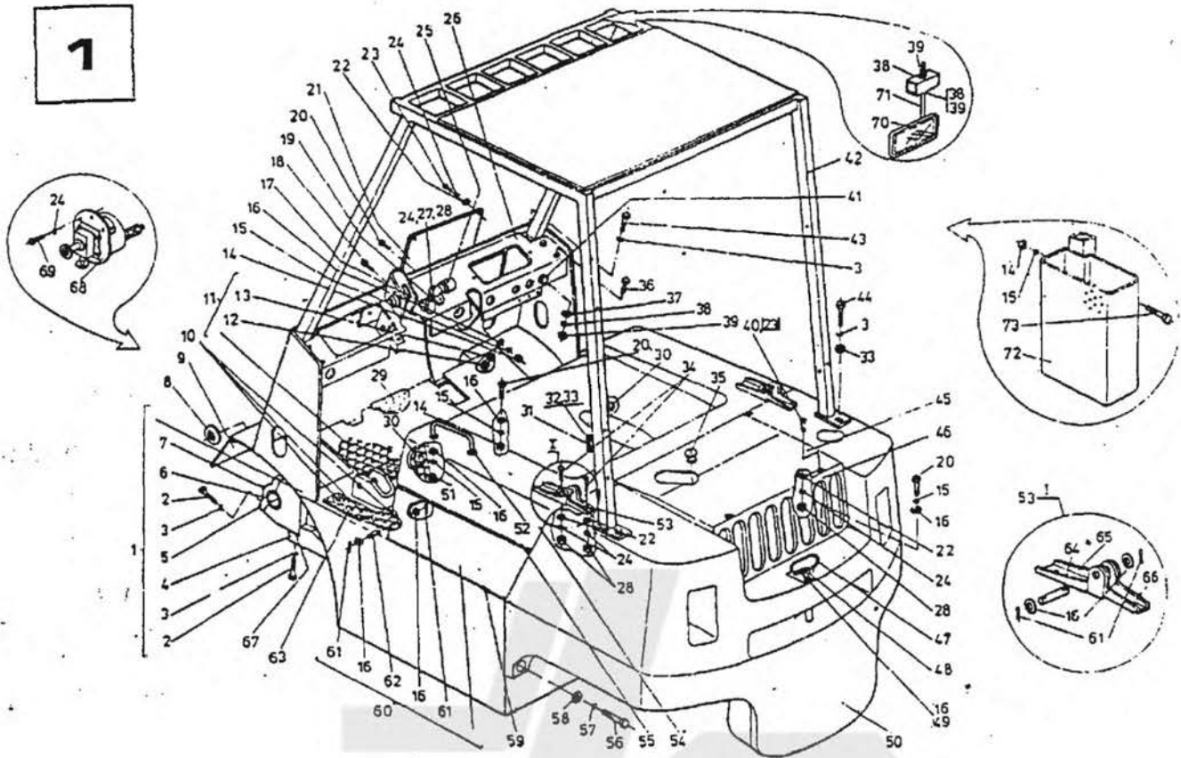
ОБЩИЙ ВИД
