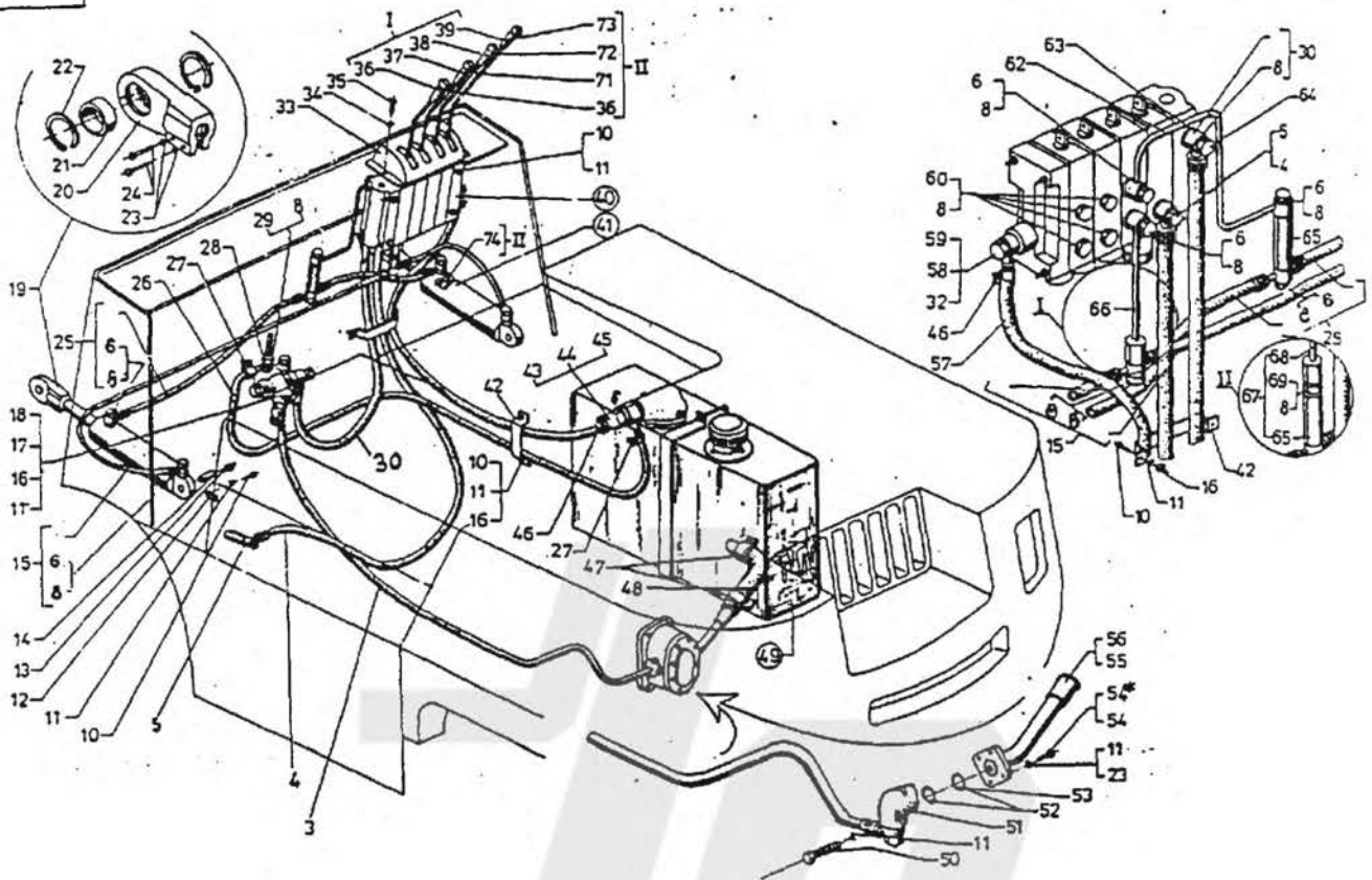
ГИДРАВЛИЧЕСКАЯ СИСТЕМА
