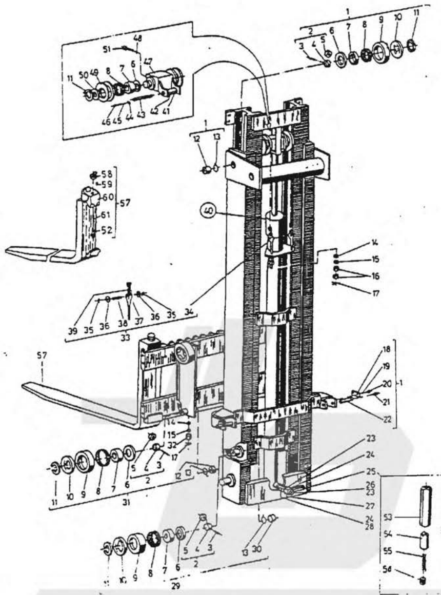
ПОДЪЕМНОЕ УСТРОЙСТВО С КЛЫКОМ ВИЛ (в сборе)
