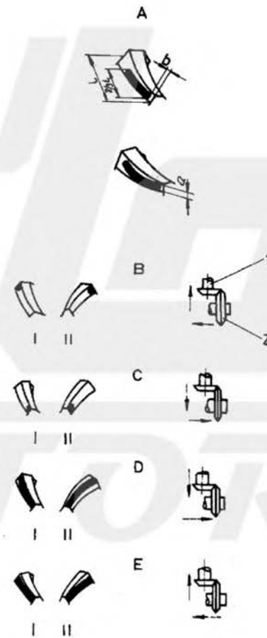
Рис.42 Регулировка зацепления конической ведущей шестерни и конической коронной шестерни
