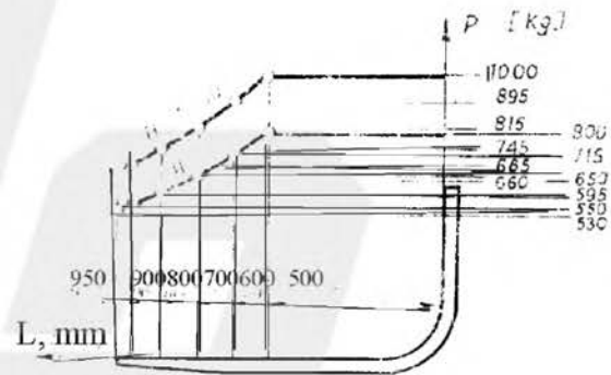
Рис. 2а Диаграмма нагрузки для погрузчиков с высотой подъема 4500 мм
