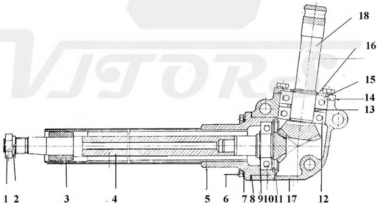
Рис. 11 Рулевая колонка
