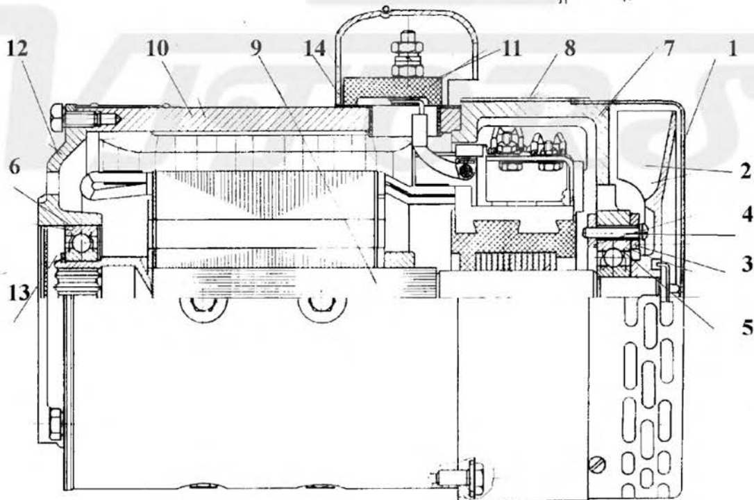
Рис. 34 Насосный электродвигатель EC 6,5/7,5/28
