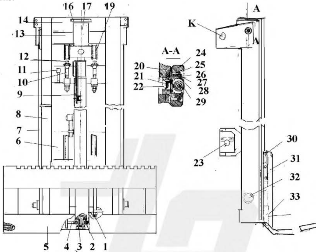
Рис. 12 Грузоподъемное устройство двухмачтовое
