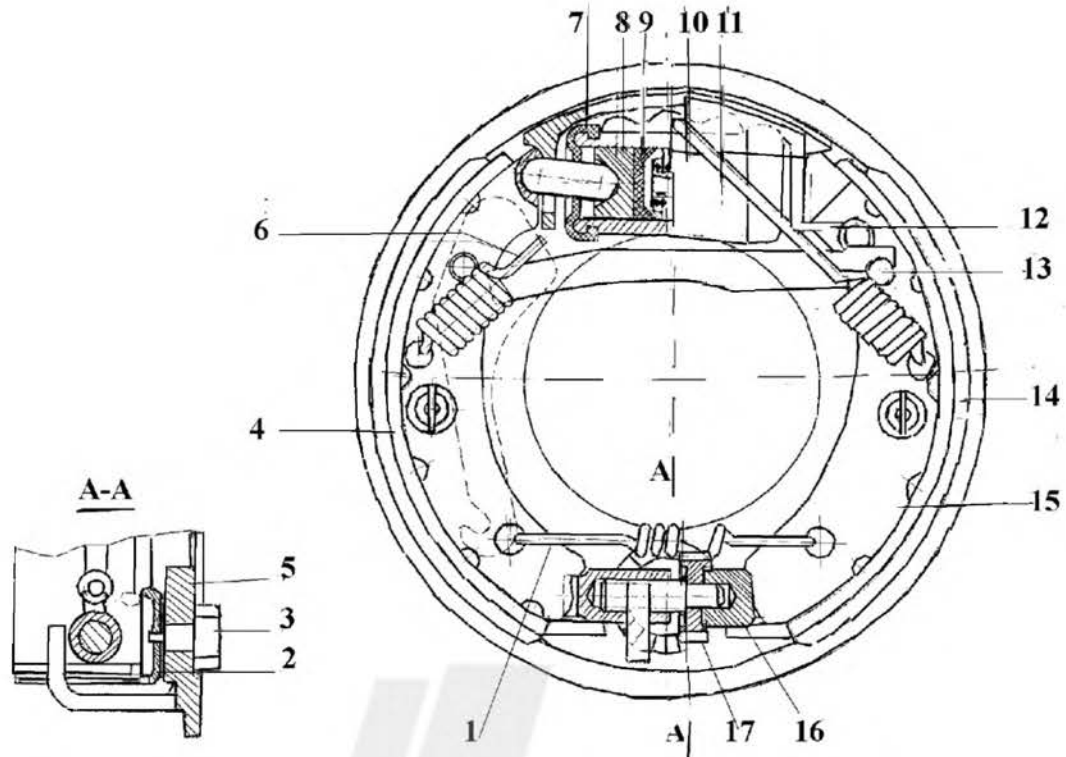
Рис. 8 Сервотормоз
