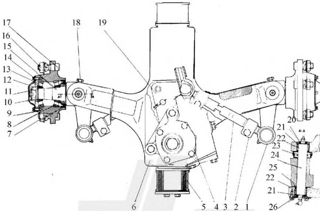
Рис.4 Управляемый мост
