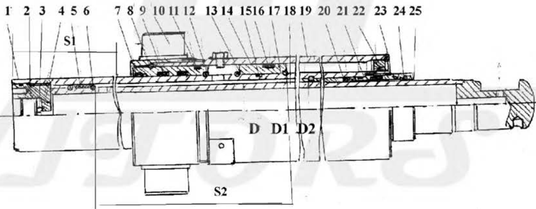
Рис. 26 Двухступенчатый телескопический цилиндр подъема
