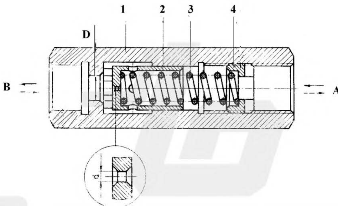
Рис. 22 Нерегулируемый дроссель ДН 12 (1,7X7,2)
