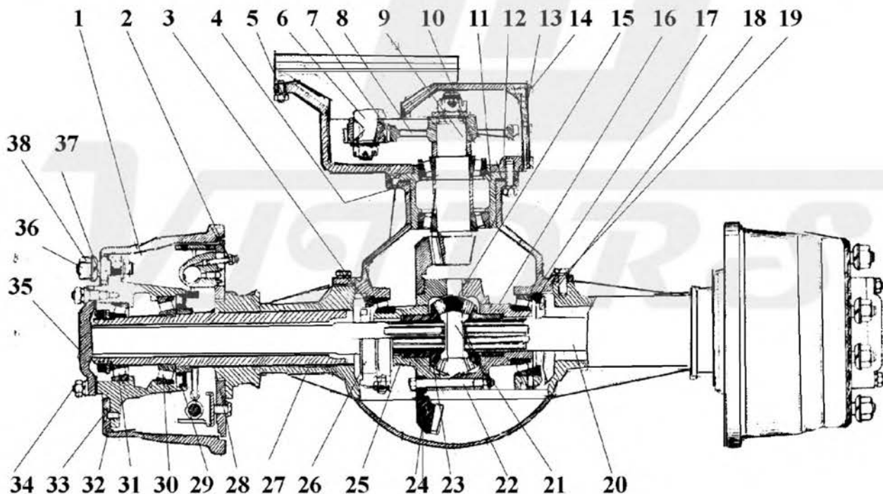
Рис.3 Трансмиссия
