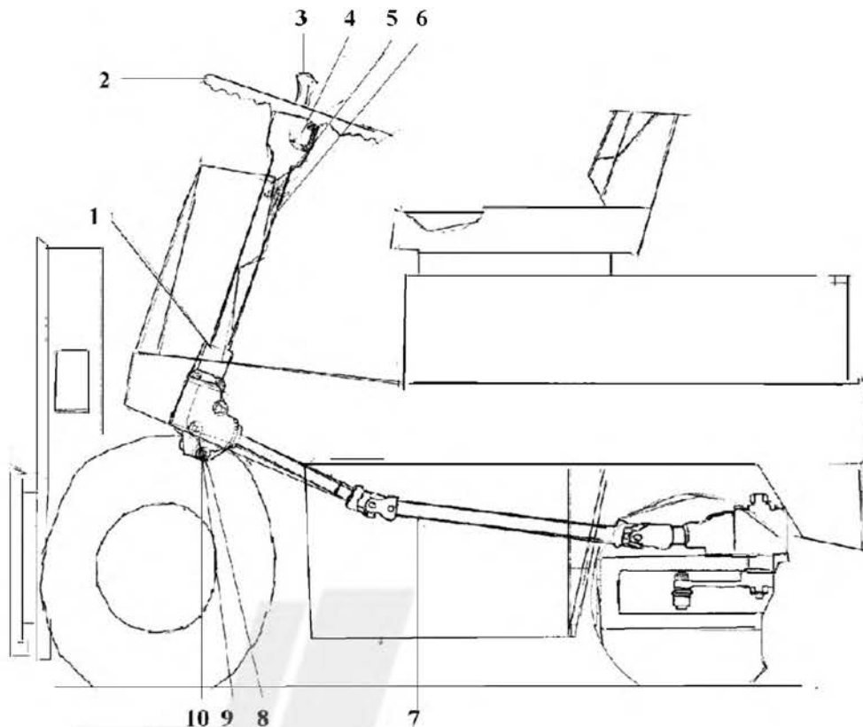
Рис. 10 Устройство управления
