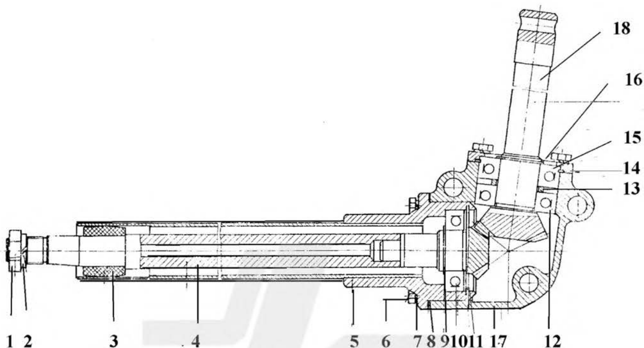
Рис. 11 Рулевая колонка
