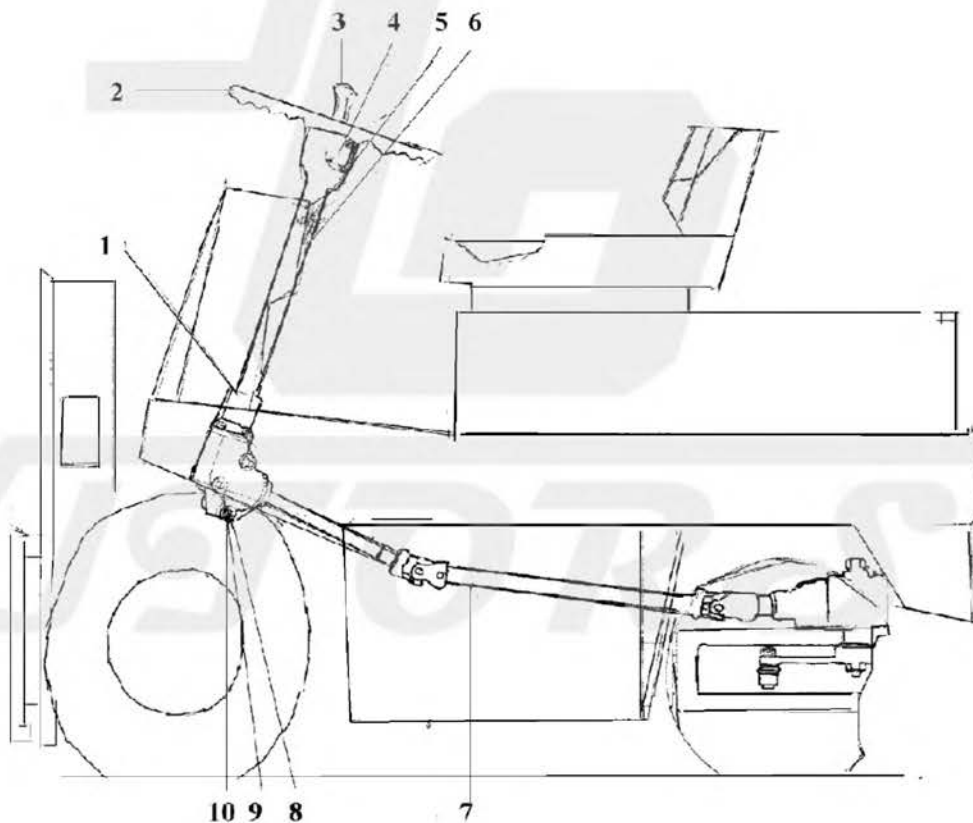
Рис. 10 Устройство управления
