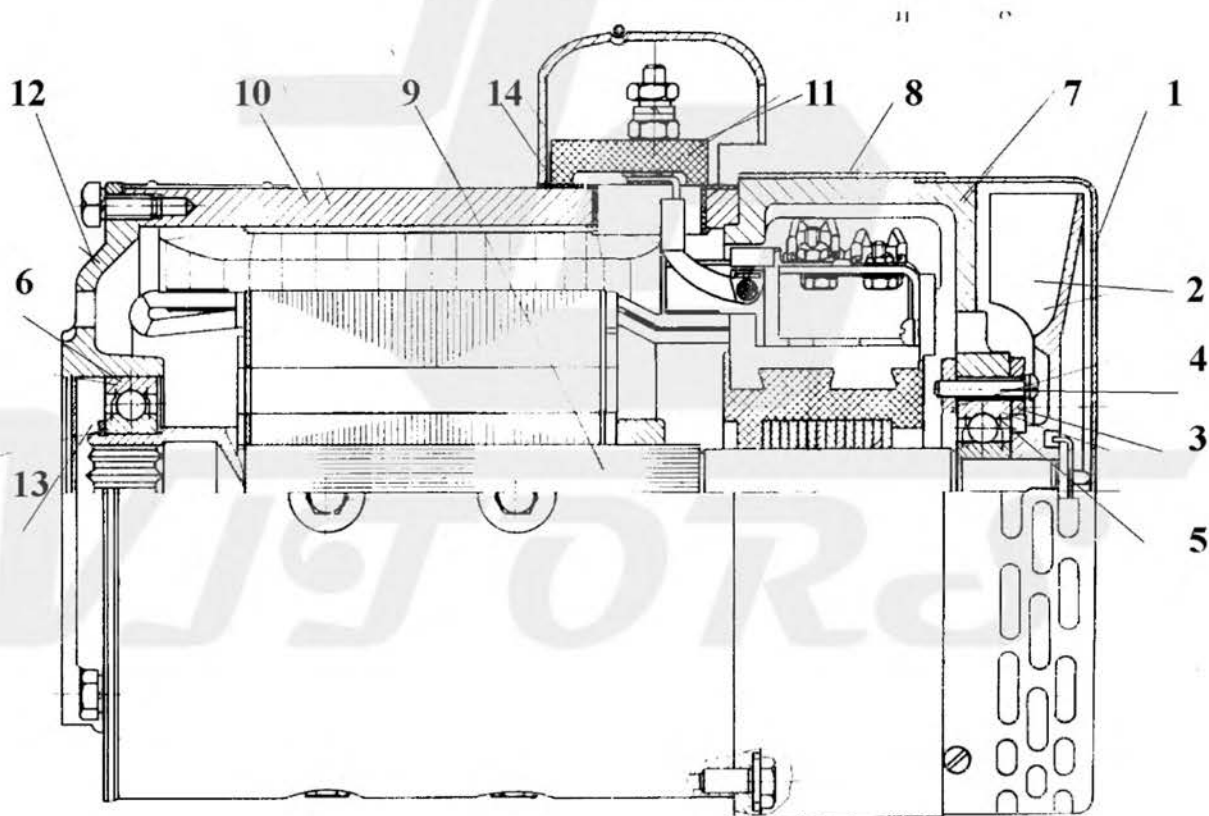
Рис. 28 Насосный электродвигатель EC 6,5/7,5/28
