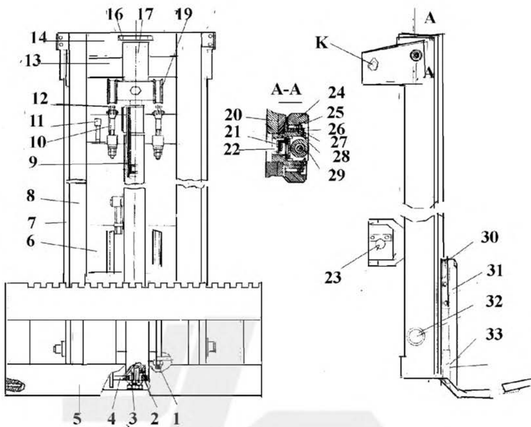
Рис. 12 Грузоподъемное устройство
